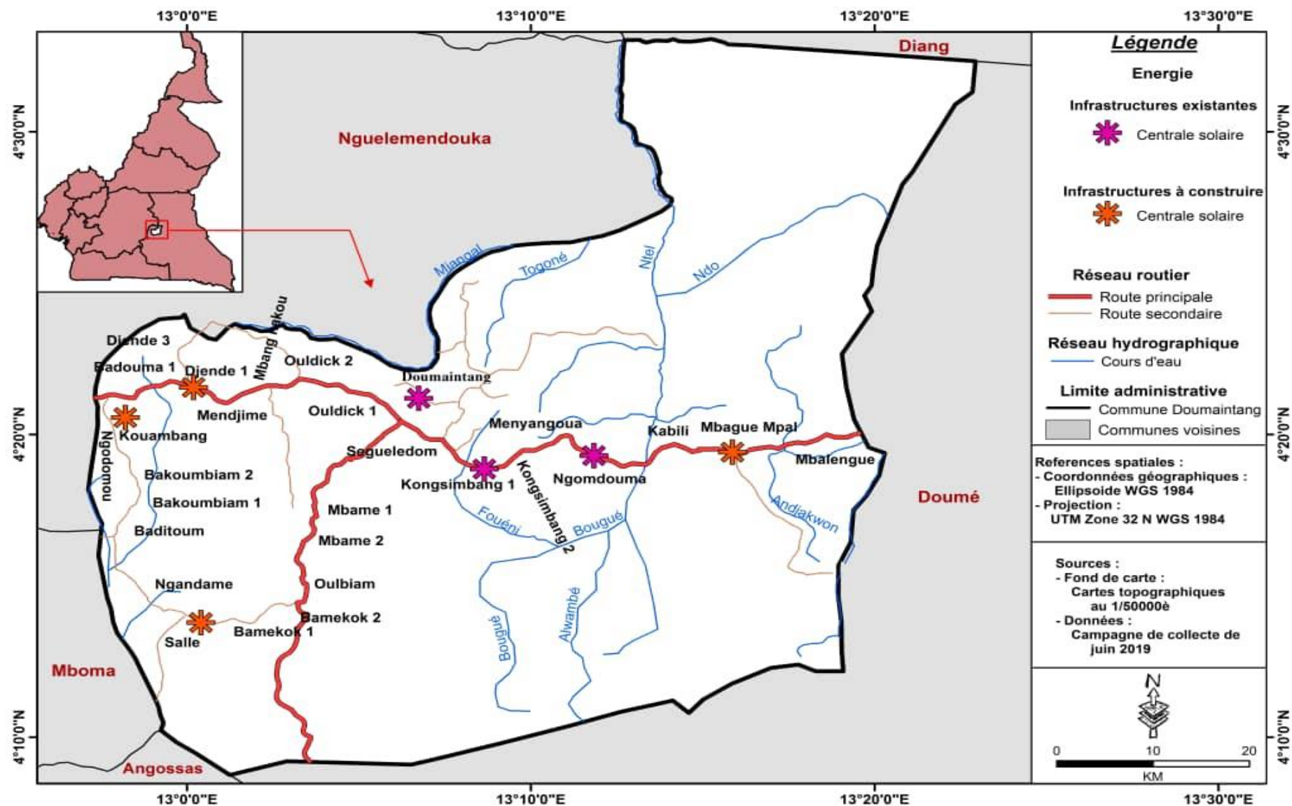
Carte 29 : Carte spatiale du secteur de l'énergie : centrale solaire à construire
