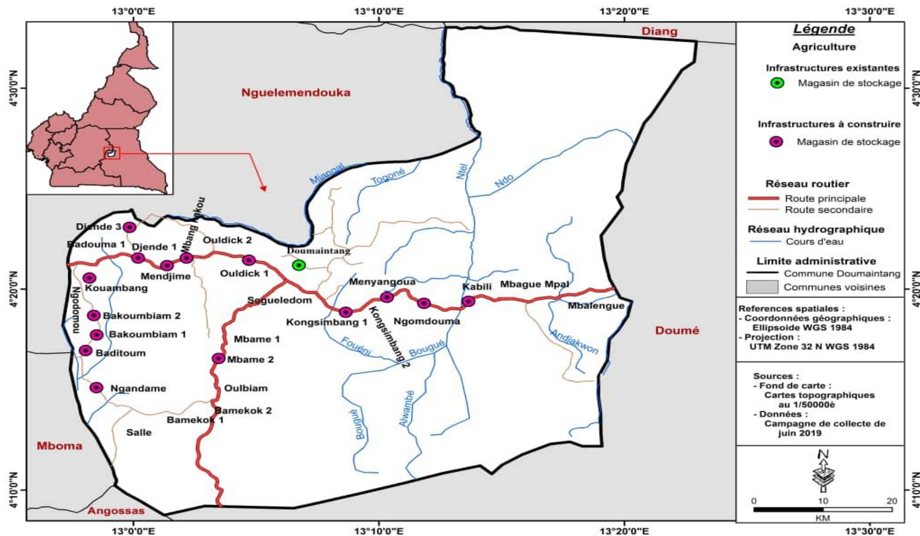
Carte 15 : carte de planification spatiale du secteur Agriculture : magasin de stockage à construire
