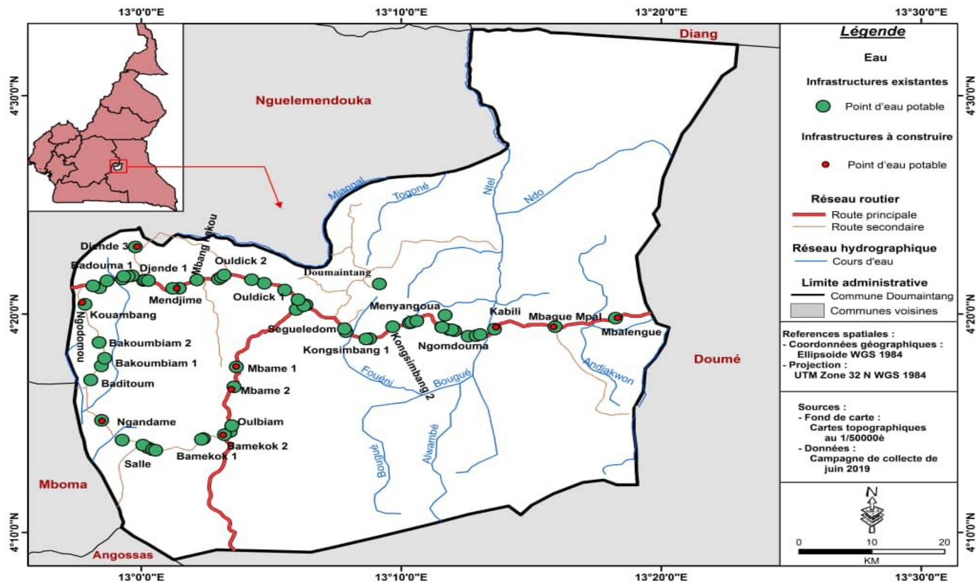
Carte 28 : Carte spatiale du secteur de l'eau : forage et puits aménagés à construire
