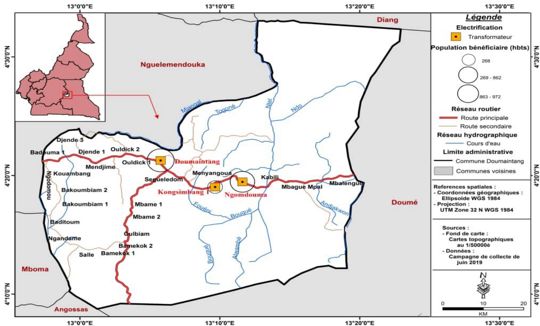
Carte 8 : Carte d'électrification de la commune de Doumaintang
